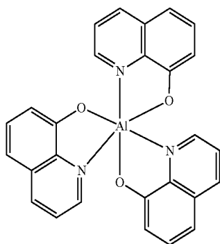
Alq 3
