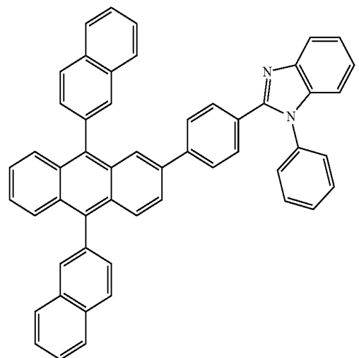
ET1
